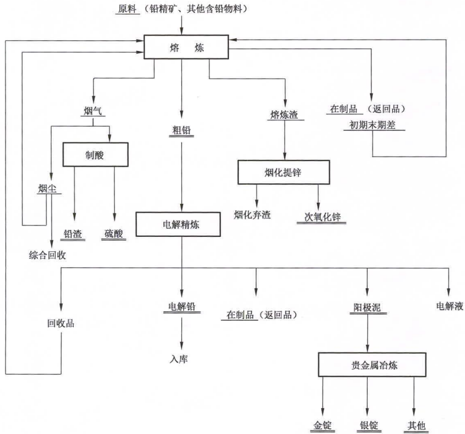
图 3 冶炼物料流程图
