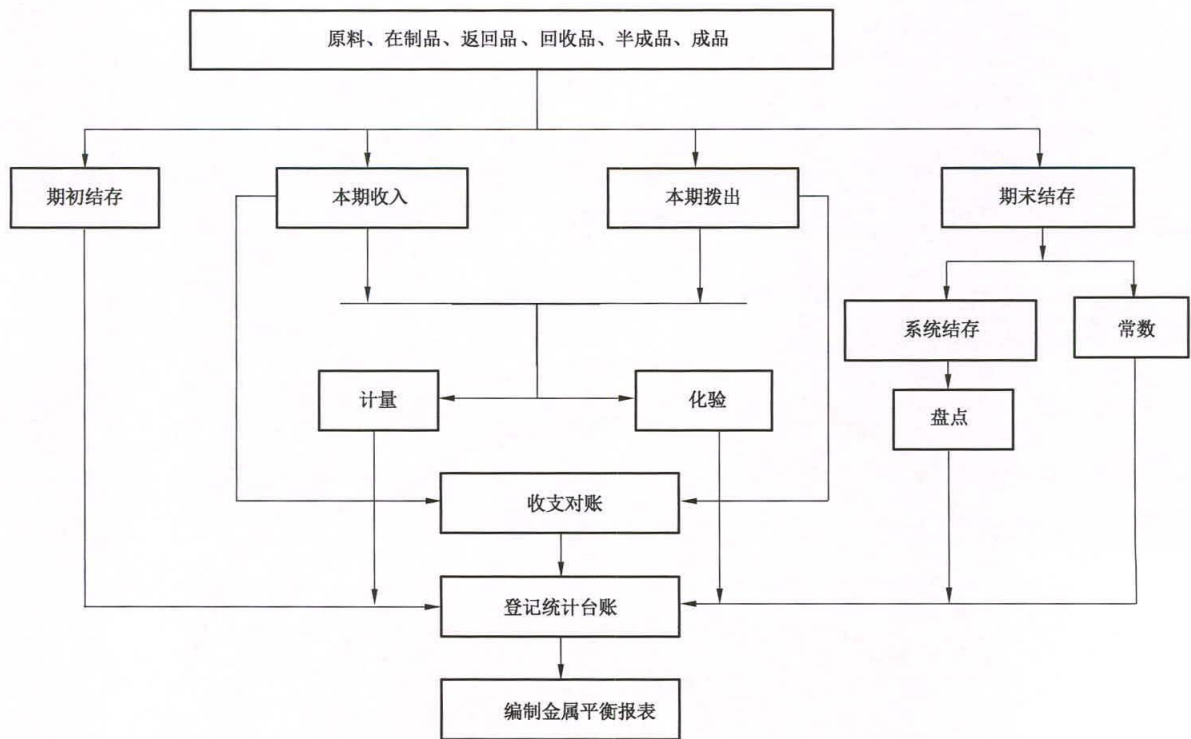
图 4 金属平衡表编程序图
